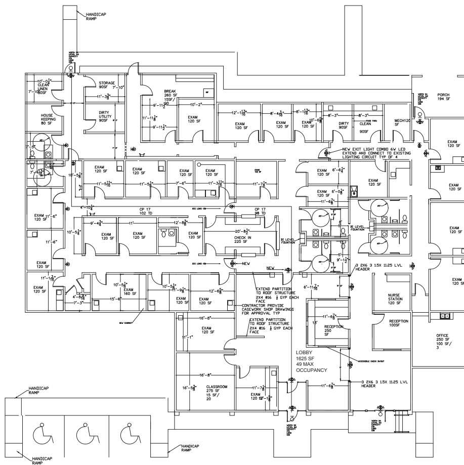
PLAN SCALE: 1/8"=1'
