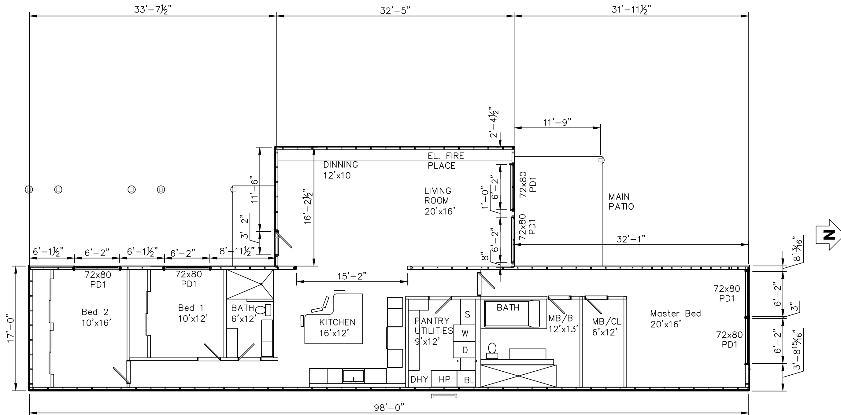
FLOOR PLAN SCALE: 1/8" = 1'-0"
